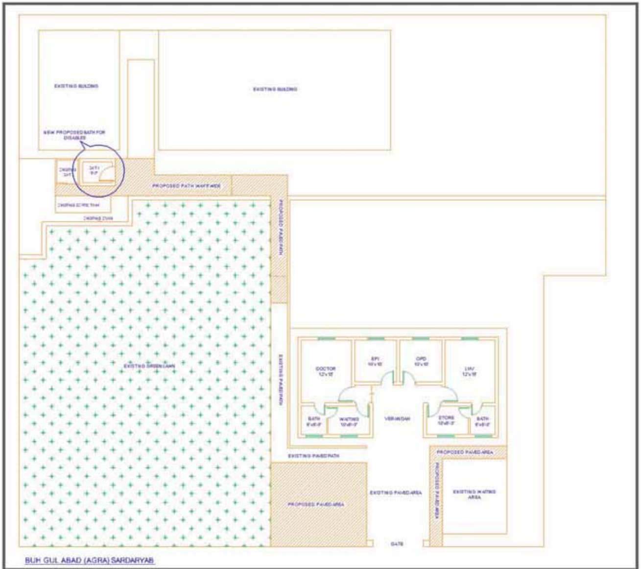
▣ Grundriss der Gesundheitsstation
